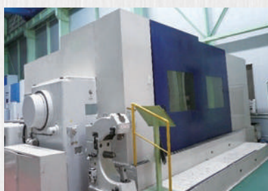
カバー w5000xL2500xH2500 t2.3(SEHC)
